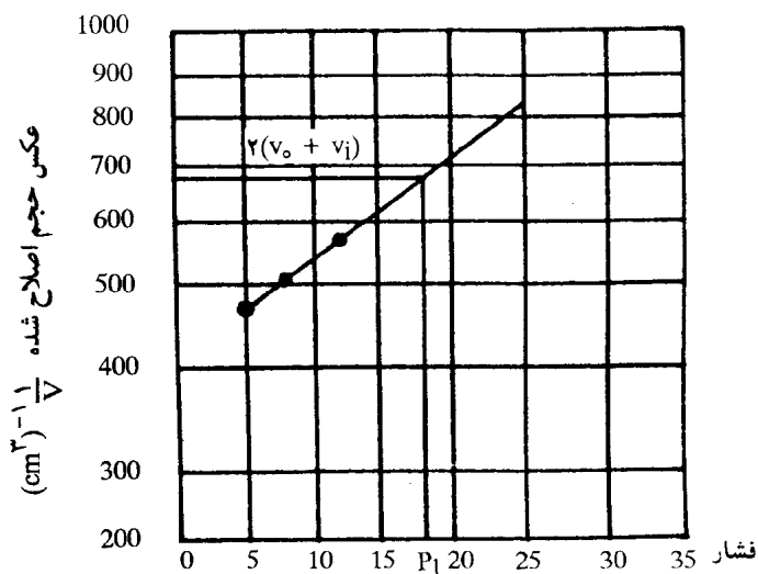
شکل شماره (۴-۴) - محاسبه فشار حدی با استفاده از نمودار \frac{1}{V} بر حسب P
